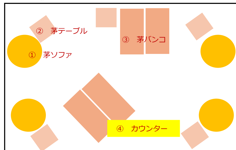
【配置例】※横6m×縦3.5mを想定した場合
