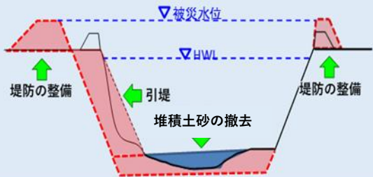
＜改良復旧イメージ断面図＞
