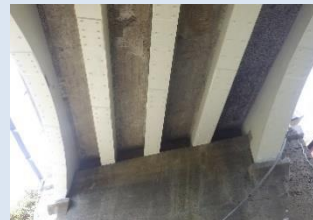
【橋りょう】モダン橋(阿蘇市)の補修
