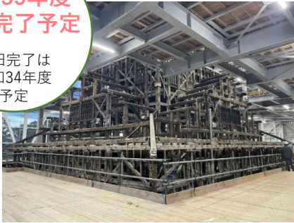
宇土櫓解体工事の様子
