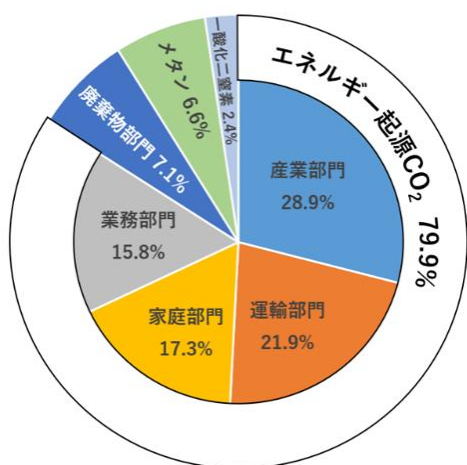
図2-1-2 温室効果ガス排出量の内訳 (部門別、2023年度)
