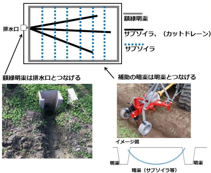
サブソイラ ほ場の耕盤の破碎や簡易な暗渠を施工する機械
