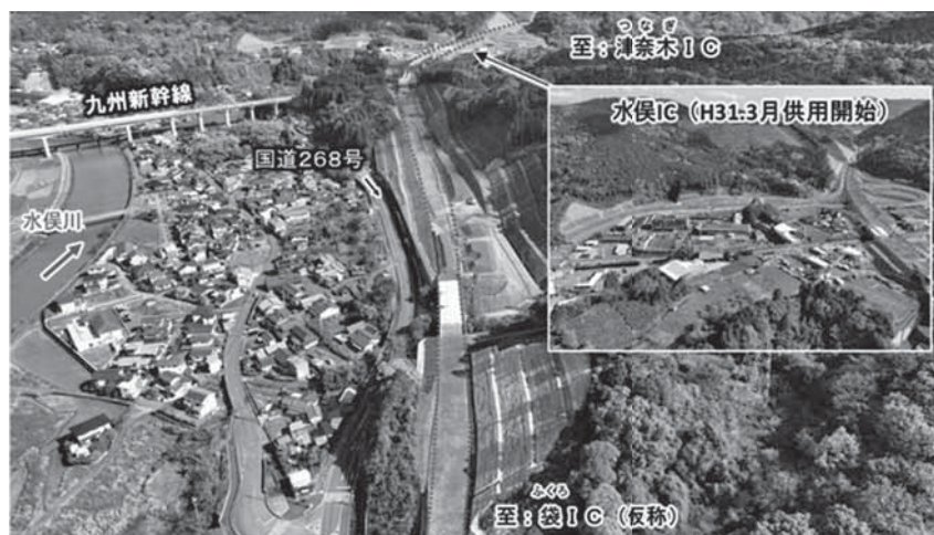
芦北出水道路の整備状況 <南九州西回り自動車道整備>
