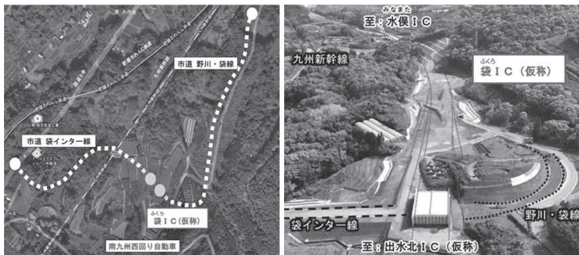
袋 I C（仮称）付近道路の整備状況 <袋インター関連道路改良事業>
